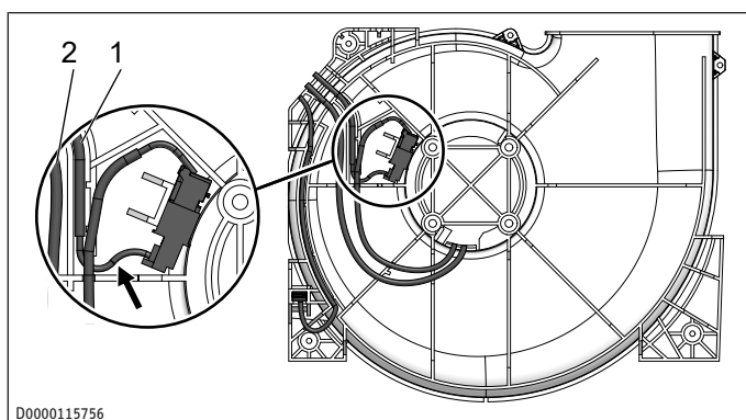
1 Fan power cable 2 Fan control cable
