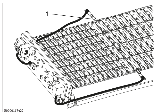
1 Sistema di sicurezza
