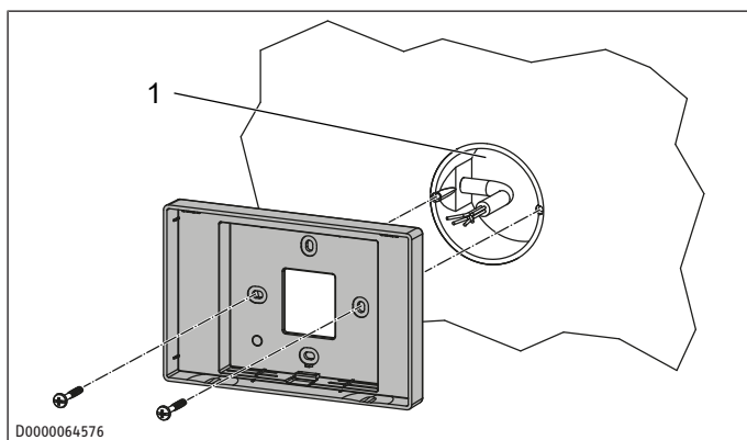
1 Flush box
