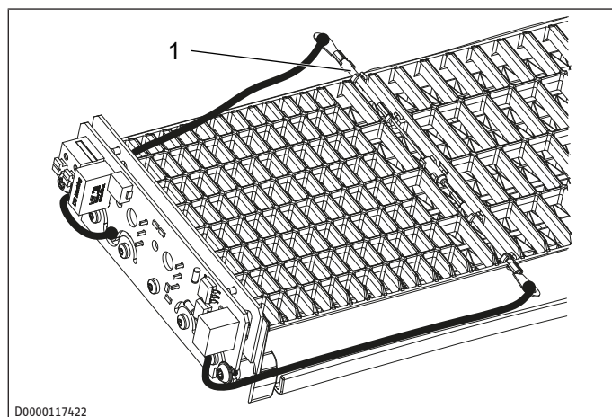
1 biztonsági modul
