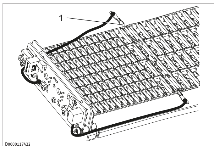
1 Bezpečnostná konštrukčná skupina
