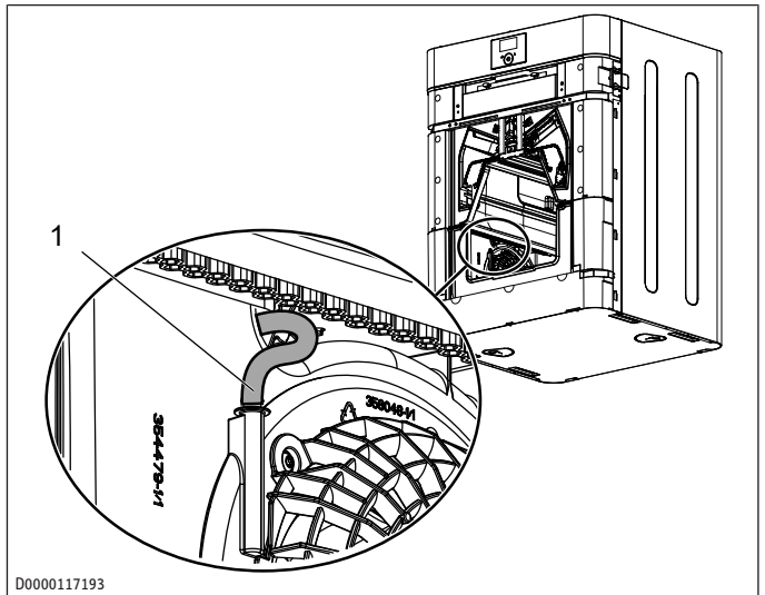
1 Drukslang
