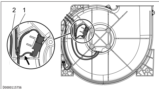
1 Netsnoer van de ventilator 2 Stuurkabel van de ventilator
