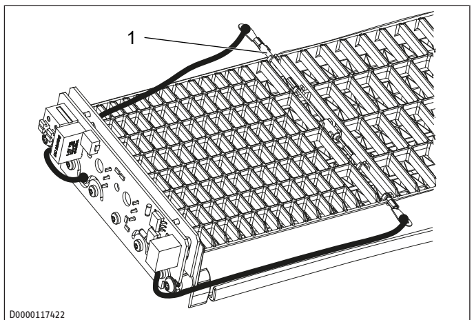
1 veiligheidsmodule
