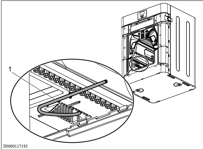
1 Drukslanghouder
