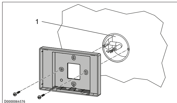
1 Scatola da incasso
