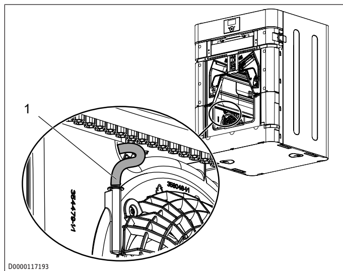
1 Tuyau antivibratoire
