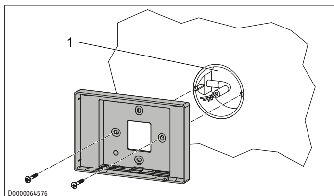
1 Puszka podtynkowa
